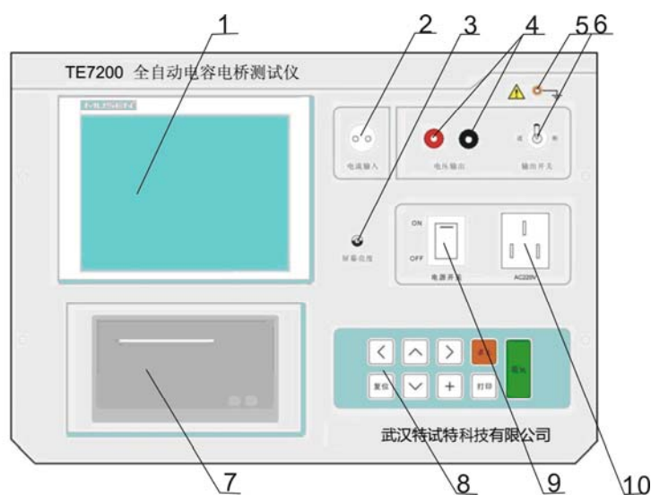
图2 仪器面板
