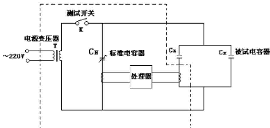
图1 电容电桥工作原理图
